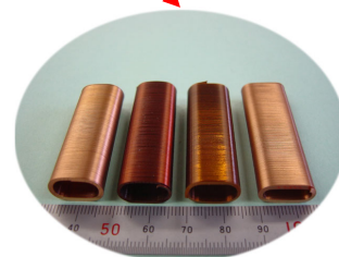
扁平线椭圆空心H形线圈
